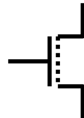
Explizite Darstellung, daß Kanal erst gebildet werden muß (positive Schwelle, 'normally Off', Enhancement-Typ)
